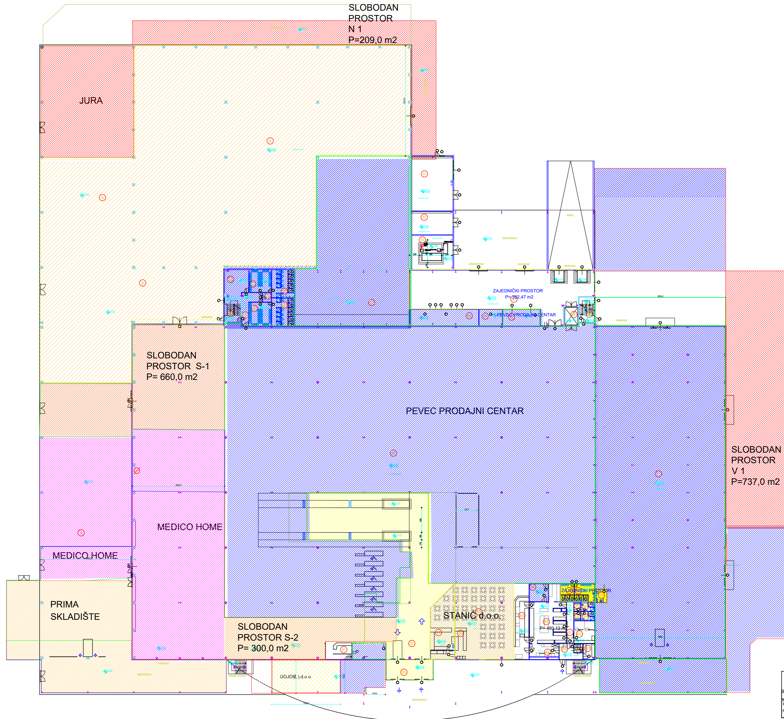
TLOCRT PRIZEMLJA
